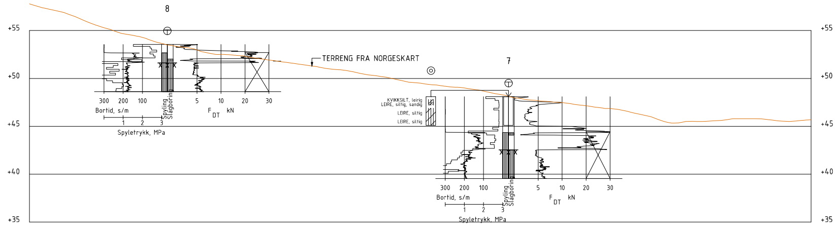
Profil E-E
