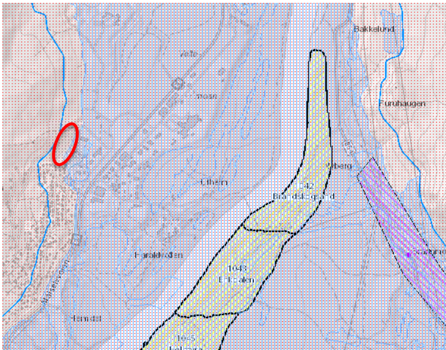
Figur 4-2: Registrerte faresoner for kvikkleireskred [6]. De gule sonene viser utløsningsområder, det skraverete mørk lilla feltet viser et kvikkleireområde og det lys lilla feltet viser området som er kartlagt for store naturlige områdeskred.
